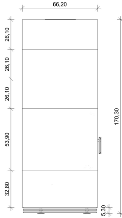
Ansicht linke Seite
